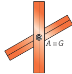
Equilibrio indifferente
