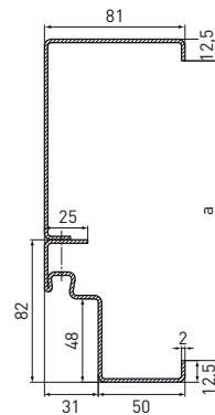
EZG avec contre huisserie 81 mm
