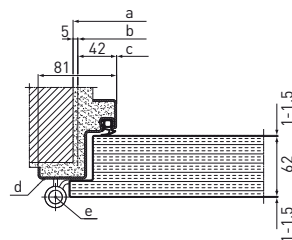
Coupe horizontale EI 2 30-2
