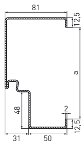
BZG type 1 pose entre murs
