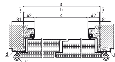
Coupe horizontale EI 2 30-2
