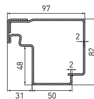
Cadre applique »Suisse« type 3 rempli en usine, pose contre le mur
