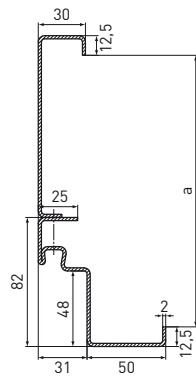
EZG avec contre huisserie 30 mm
