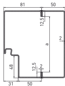
BZG type 2 pose entre murs, cadre élargi
