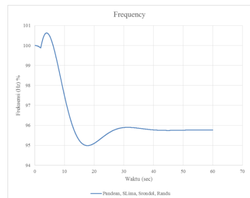
Gambar 4. 3 Pergerakan Frekuensi Saat Generator GTG 1.3 Outage dari system dengan mekanisme Load Shedding tahap 2
