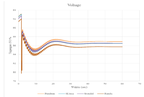
Gambar 4.6 Pergerakan Tegangan kondisi Generator 2 KL Outage dari Sistem dengan Mekanisme Load Shedding Tahap 3
