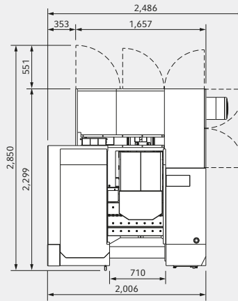
LASERTEC 50
