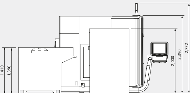
LASERTEC 50
