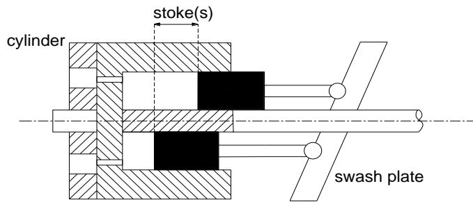
Figure1.5 Swash-plate piston motor
