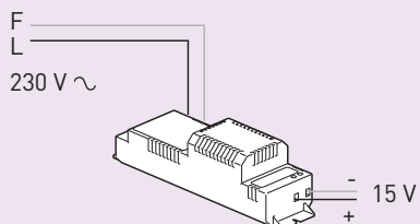
Inštalácia napájania do podlahu
