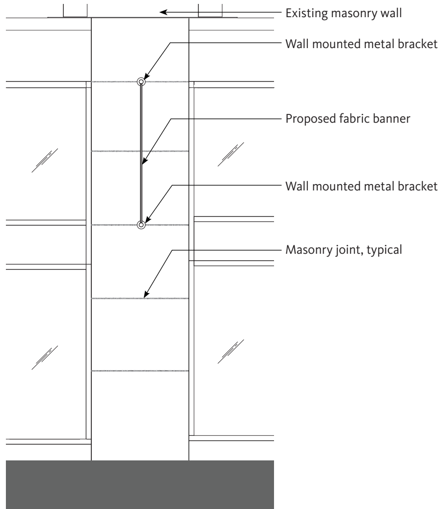
Elevation
