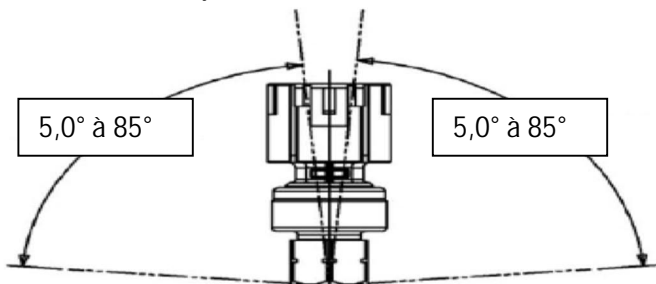
ORIENTATION DE MONTAGE PERMISE DANS TOUTE DIRECTION RELATIVE À LA POSITION VERTICALE
