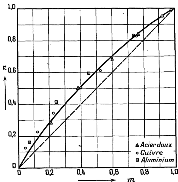
Résultats des essais de MM. Taylor et Quinney [37]; la courbe correspond à H = S^1_2 - 0,65 S^2_2 , la droite pointillée à l'hypothèse de Saint-Venant.
