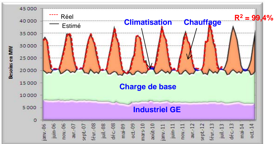
Modèle de prévision des besoins en puissance
