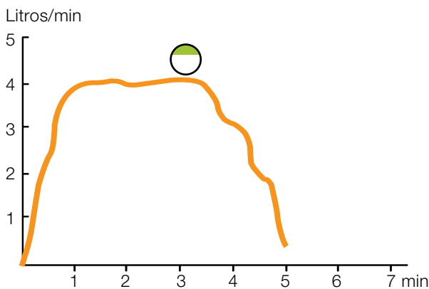
a) Patrón de flujo de leche de una vaca bien estimulada
