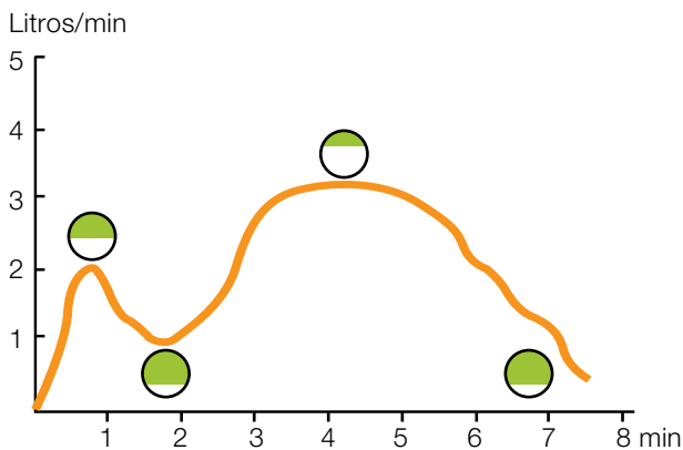
b) Patrón bimodal de flujo de leche de una vaca mal estimulada. El tiempo de ordeño es mayor.
