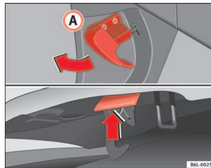
Fig. 120 Gancho apertura capó motor.
