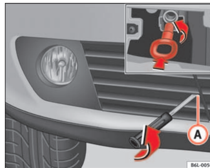
Fig. 161 Argolla de remolque delantera
