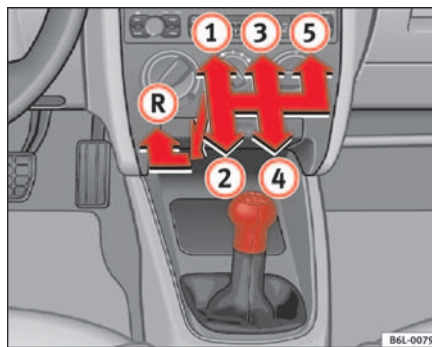
Fig. 95 Consola Central: esquema de un cambio manual de 5 marchas
