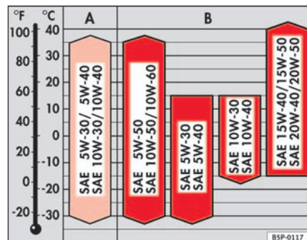
Fig. 121 Tipos de aceite de acuerdo a la temperatura
