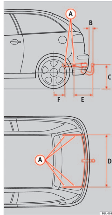
Fig. 118 Puntos de fijación del dispositivo de remolque
