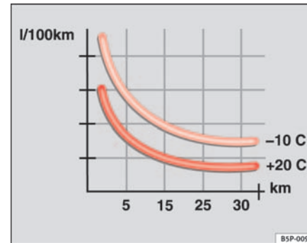
Fig. 117 Consumo de combustible (l/100 km) a dos temperaturas ambiente
