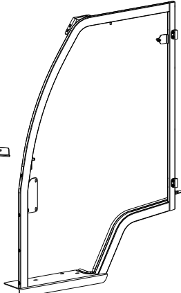
SIDE FRAME LEFT P/N: 8SV-GC17909L-G1
