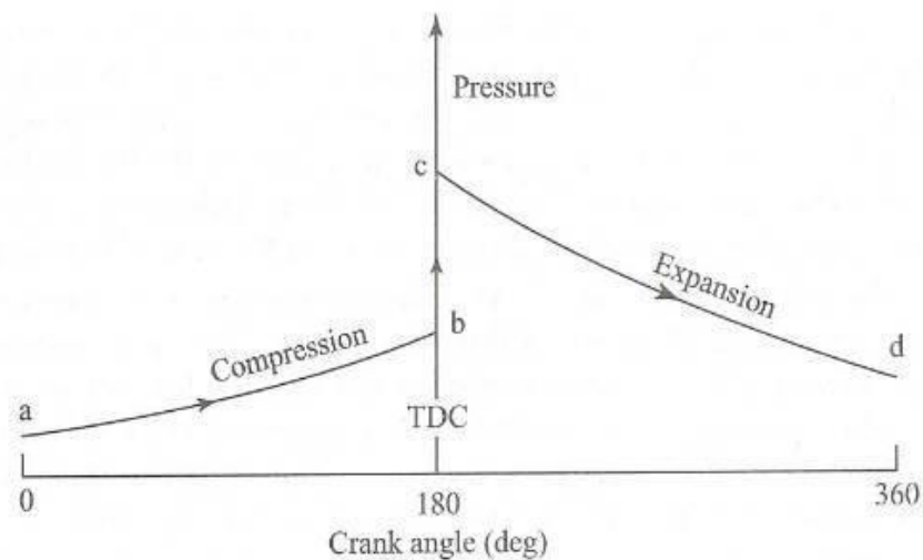
Actual p-θ diagram
