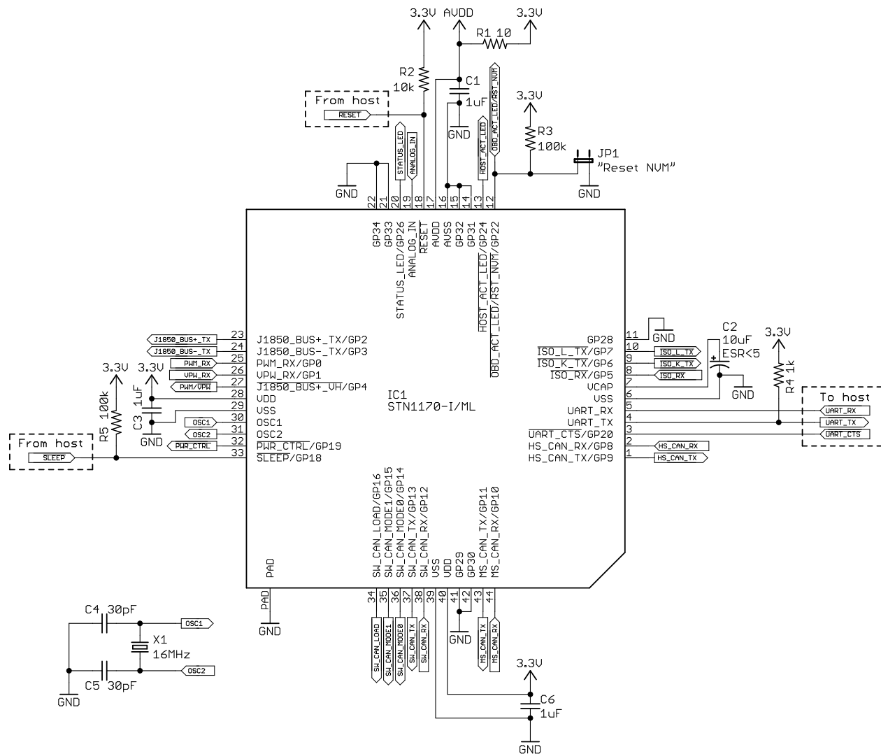
Figure 2 – STN1170 IC
