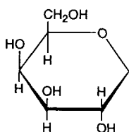
1,5-Anhydro-D-galactitol
