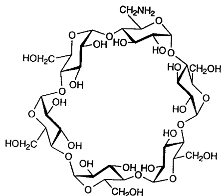
6 1 -Amino-6 1 -deoxycyclomaltohexaose
