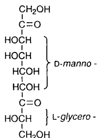
L-glycero-D-manno-Nono-2,7-diulose
