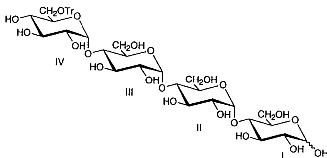
6 IV -O-Tritylmaltotetraose
