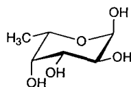
\alpha -L-Fucopyranose
