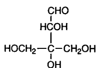
D-Apiose (Api)
