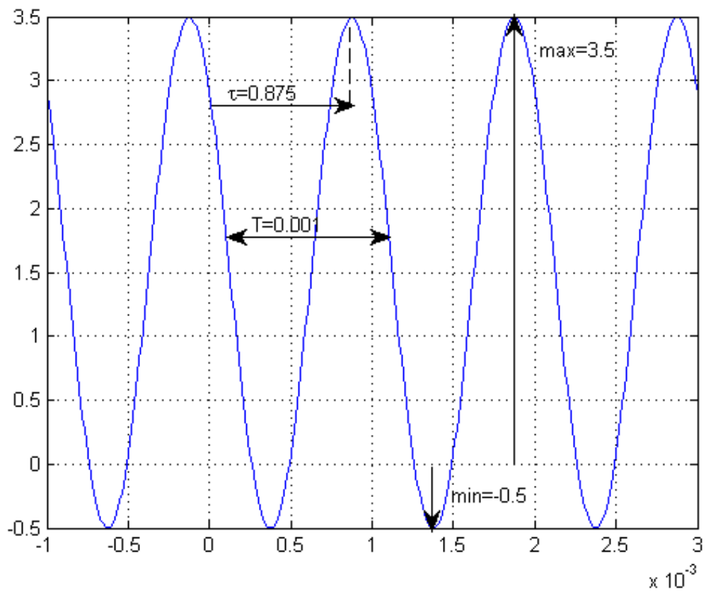
FIGURE C.1 – Signal sinusoïdal ajouté à une composante continue.
