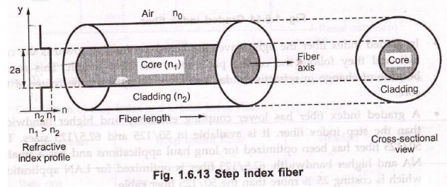
Fig. 1.6.13 Step index fiber
