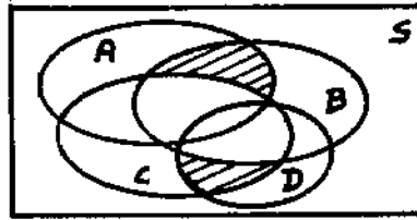
(d) (A \cap B \cap \bar{C}) \cup (\bar{B} \cap C \cap D)
