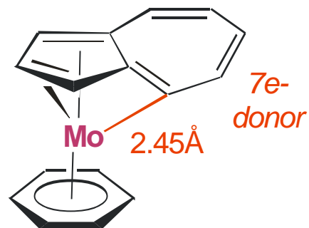
fluorenyl (-)
