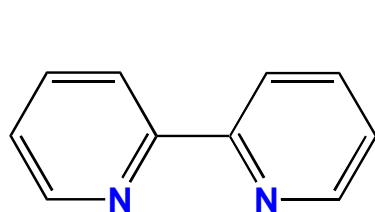
Bipy = Bipyridine
