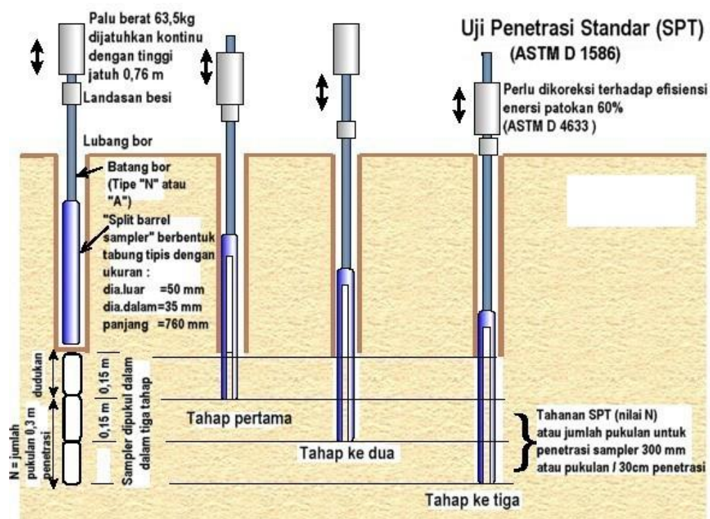
Gambar 5.6 Skema urutan uji penetrasi standar (SPT) (sumber : SNI 4153-2008)
