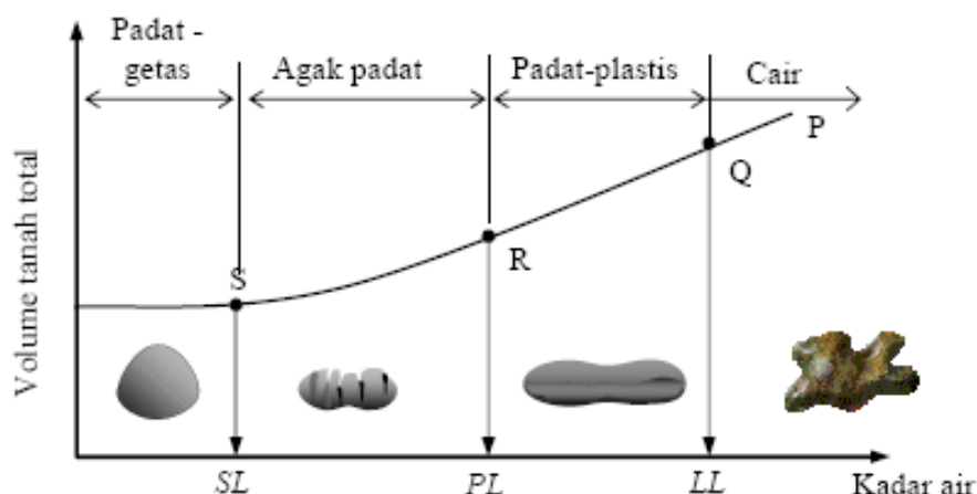
Gambar 6.4 Variasi volume dan kadar air pada Batas-batas Atterberg
