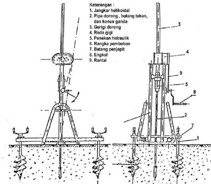
Gambar 5.4 Rangkaian alat penetrasi konus berdasarkan SNI 2827:2008
