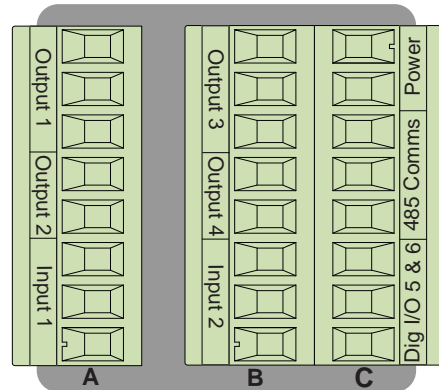
1/16 DIN PM6
