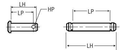
Pivot Pin
