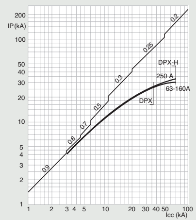
DPX 250
