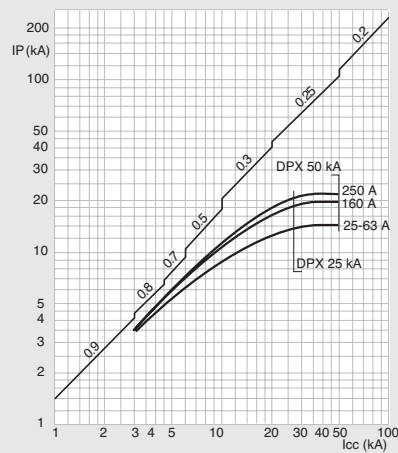
DPX 160 - 250 ER
