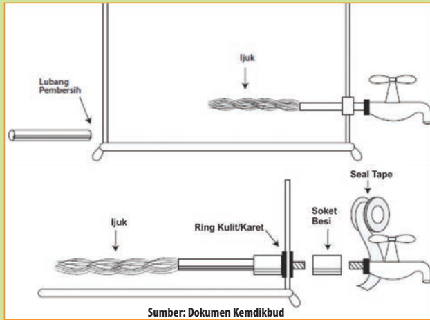
Sumber: Dokumen Kemdikbud Gambar 2.19 Pipa penyaring
