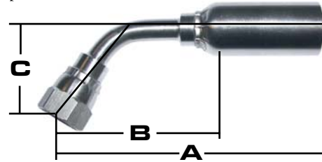
303 DIN 24° LIGHT 45°
