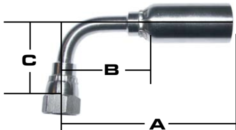
303 DIN 24° LIGHT 90°
