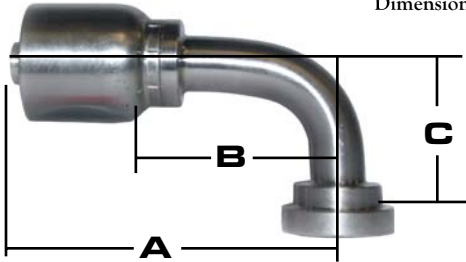
316 CODE 62 FLANGE 90°
