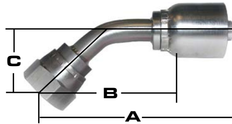
316 DIN 24° HEAVY 45°
