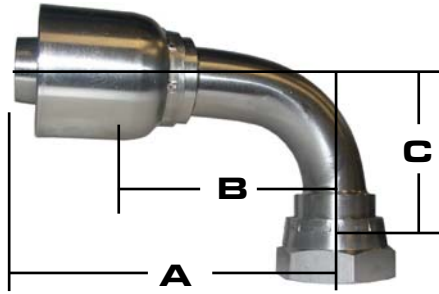
316 DIN 24° LIGHT 90°
