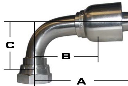
316 DIN 24° HEAVY 90°
