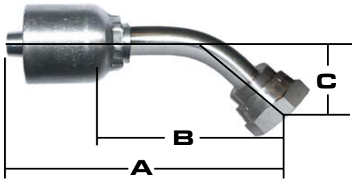
316 DIN 24° HEAVY 45°
