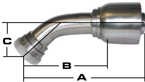
316 DIN 24° LIGHT 45°
