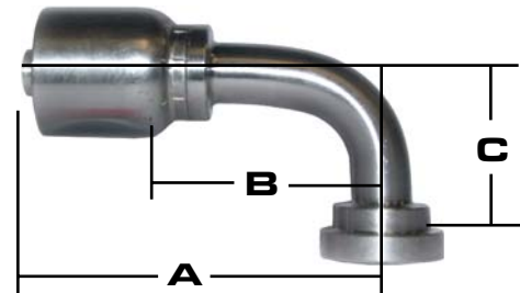
316 CODE 61 FLANGE 90°
