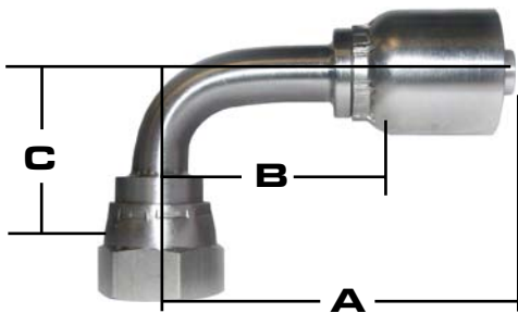
316 DIN 24° HEAVY 90°
