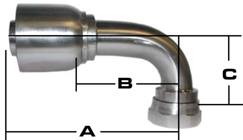
316 DIN 24° LIGHT 90°
