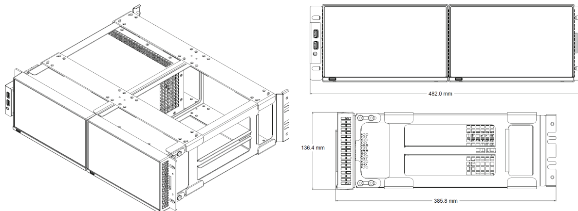
MPI2-RACK-MD
