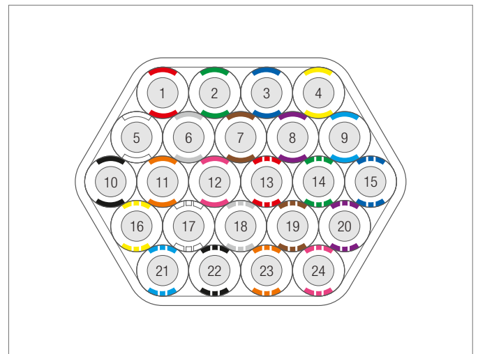
Beispiel: RAUSPEED 24x7x1,5 bzw. 24x10x2,0
