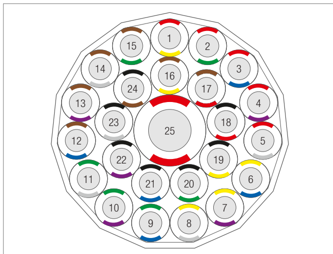
Beispiel: RAUSPEED 24x7x1,5 + 1x14x2,0
