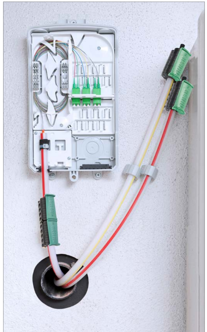
Ansicht Hausanschlussbox (AP)
