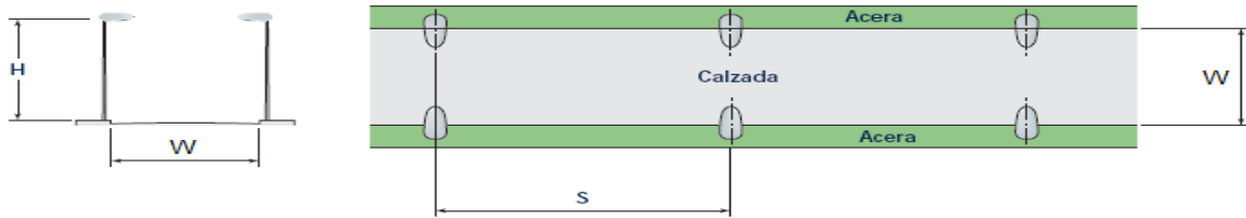
Figura 510.5.1 d. Disposición Bilateral opuesta
