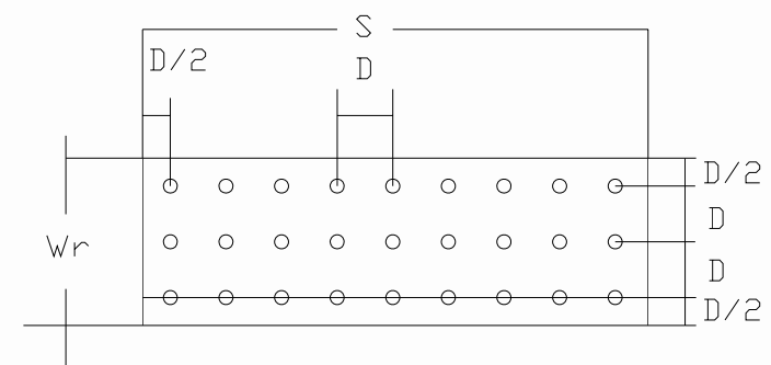
MALLA DE MEDICION PARA ILUMINANCIA CIE 140-2000 NTC 900
