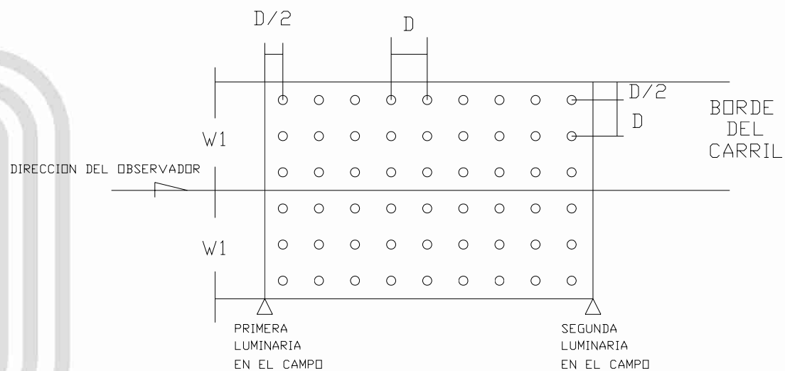
MALLA DE MEDICION PARA LUMINANCIA CIE 140-2000 NTC 900
