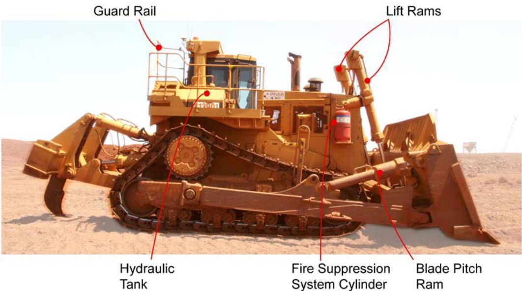
Cat D11R Right Side Profile
