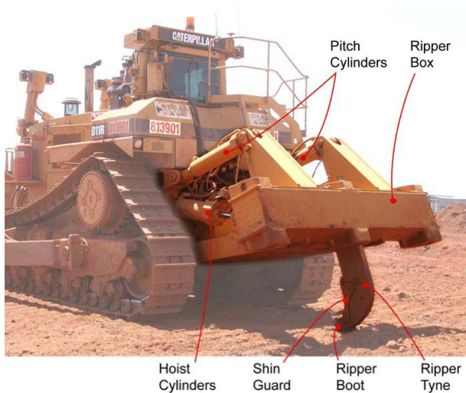
Cat D11R Rear Profile
