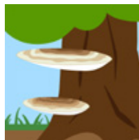
PARASITE/HARMFUL
