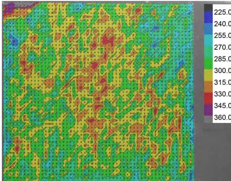
15%CF MHI Alloy 152 Hardness Range: 240-345 HV Est. Test Plane: ~305 HV
