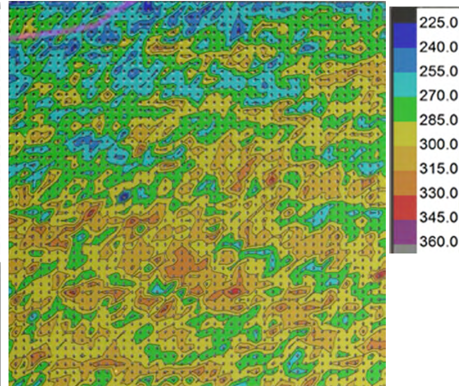
15%CF IHI Alloy 152M Hardness Range: 230-340 HV Est. Test Plane: ~300 HV
