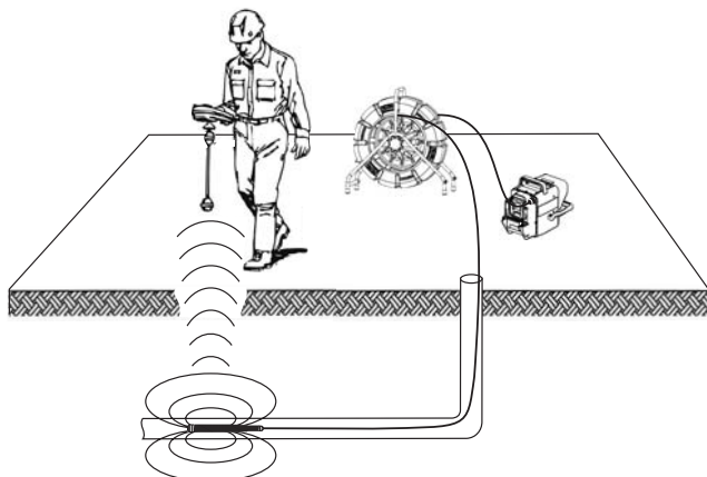
Figura 23 – Localización de la Sonda del microReel
