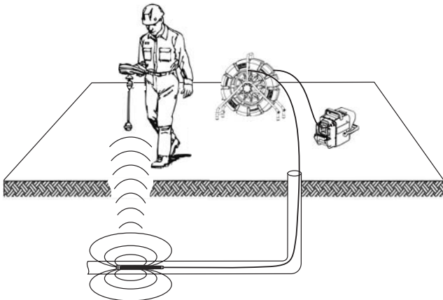
Figure 23 – Localisation de la sonde microReel
