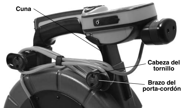
Figura 9 – Cuna y brazos del porta-cordón
