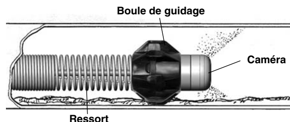
Figure 20 – Fonctionnement des boules de guidage
