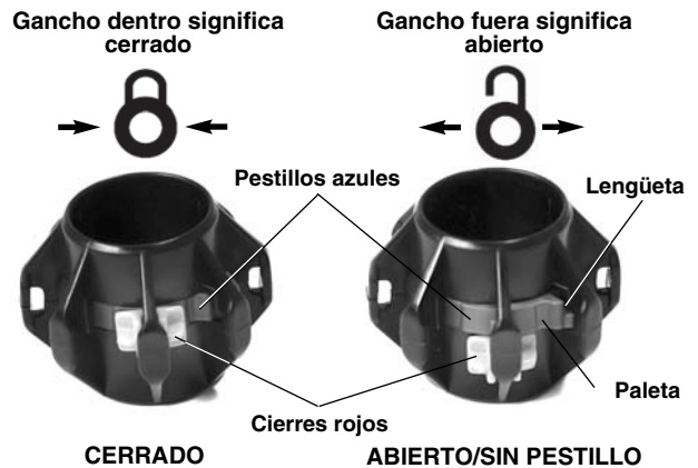
Figura 11 – Apertura y cierre de una bola-guía
