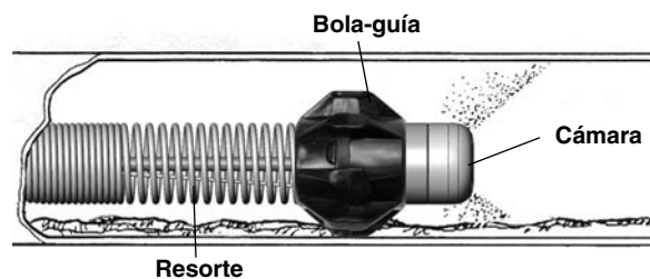
Figura 20 – Empleo de una bola-guía
