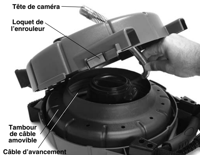
Figure 3 – Ouverture de l'enrouleur
