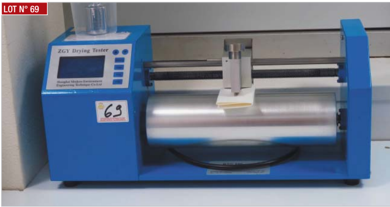
► ZCY DRYING TESTEUR BDG 660 pour évaluer le séchage des encres, année 2015 ► ZCY DRYING TESTUR BDG 660 for assessing ink drying year 2015
