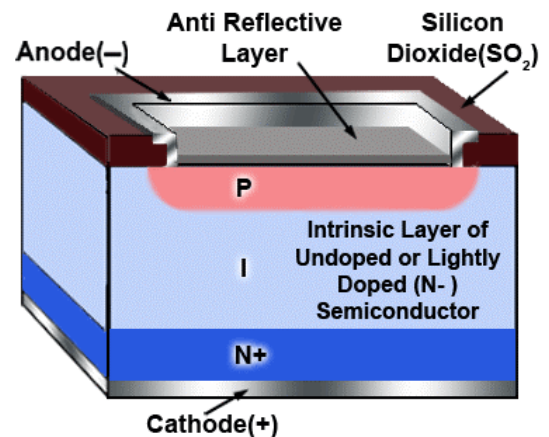
Fig. 2.7.8 PIN Photodiode
