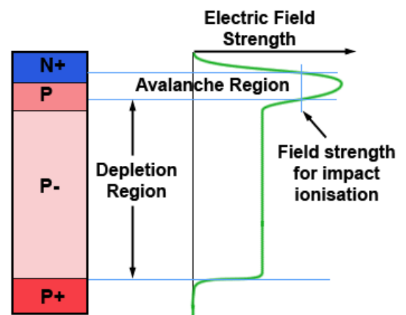
Fig 2.7.11 Impact Ionisation
