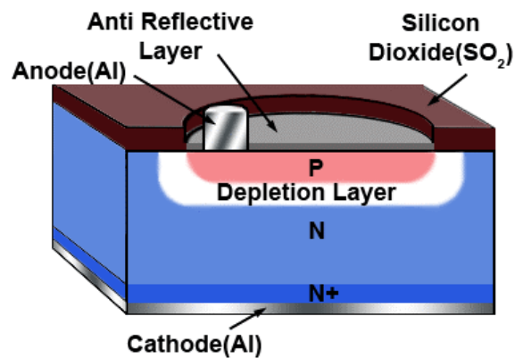
Fig. 2.7.3 Photodiode Construction
