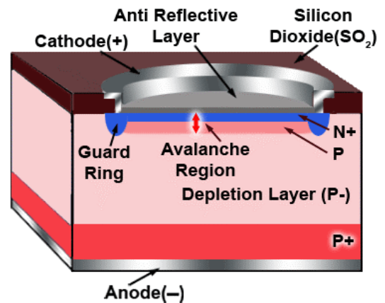
Fig. 2.7.8 The Avalanche Photodiode
