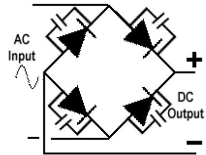
Fig 2.1.3 Spike Suppression
