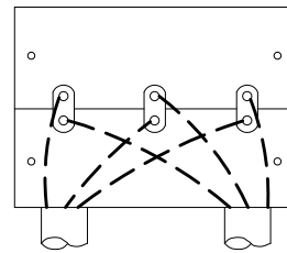
FIGURE 2 6 CABLES 2 CONDUITS
