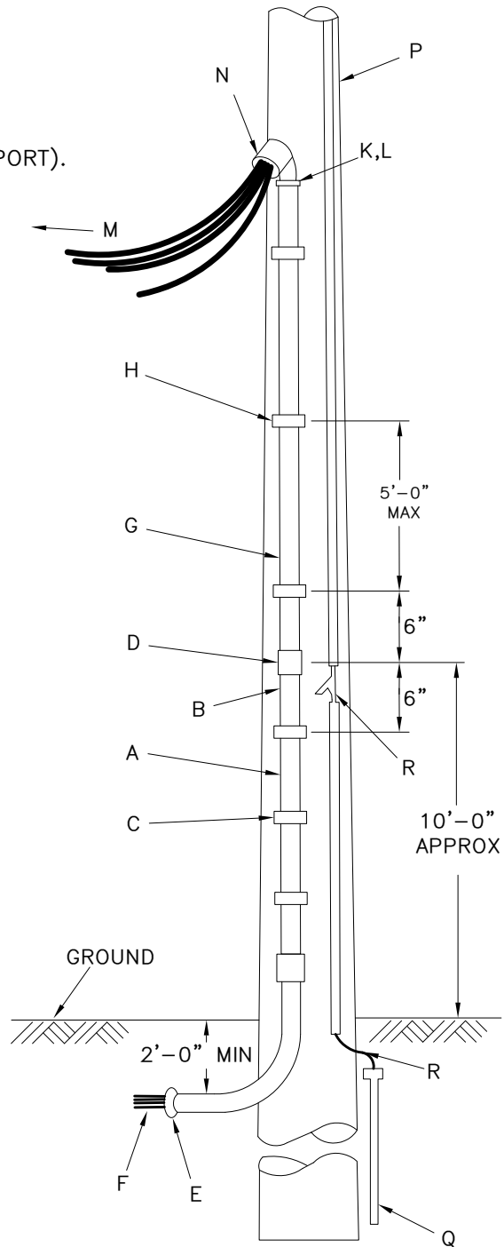
SINGLE CONDUIT RISER
