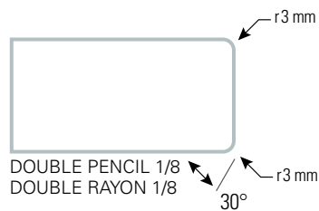
EASED BORDURE ADOUCIE
