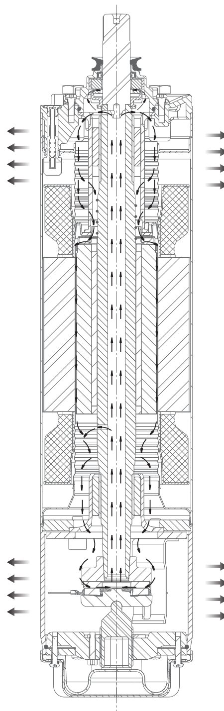
Fig. 14 MS 6000
