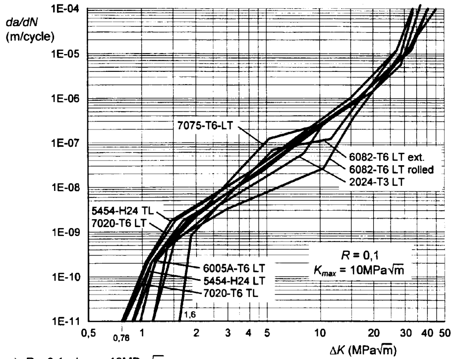
a) R = 0,1; k_{max} = 10 \text{ MPa}\sqrt{\text{m}}
