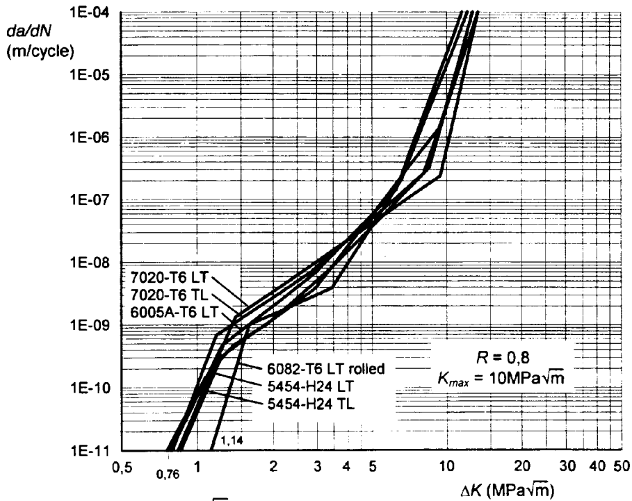
b) R = 0,8; k_{max} = 10 \text{ MPa}\sqrt{\text{m}}
