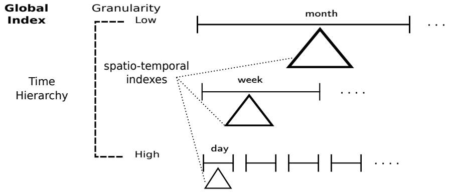
Fig. 12 ST-Hadoop spatio-temporal meta-data index
