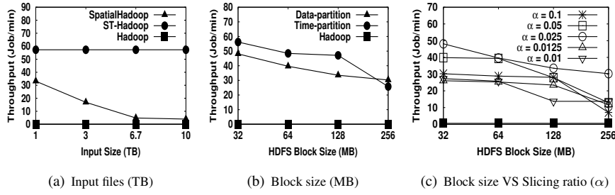
Fig. 16 Spatio-temporal Range Query
