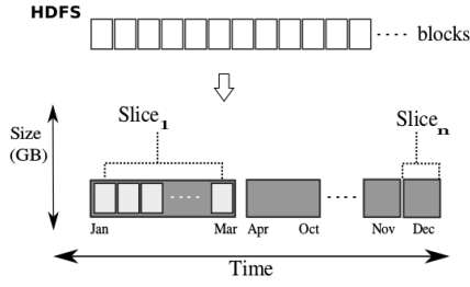
Fig. 5 Data-Slice
