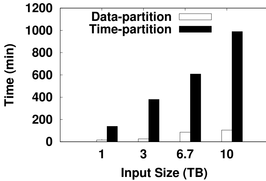
Fig. 14 Input Files
