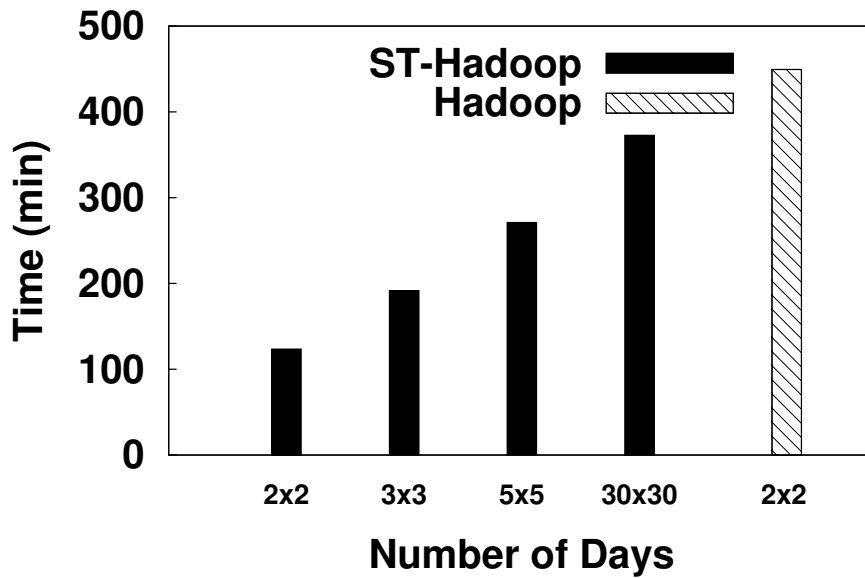
Fig. 18 Spatio-temporal Join
