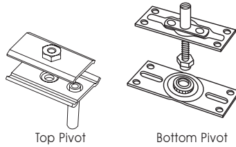
Top Pivot
