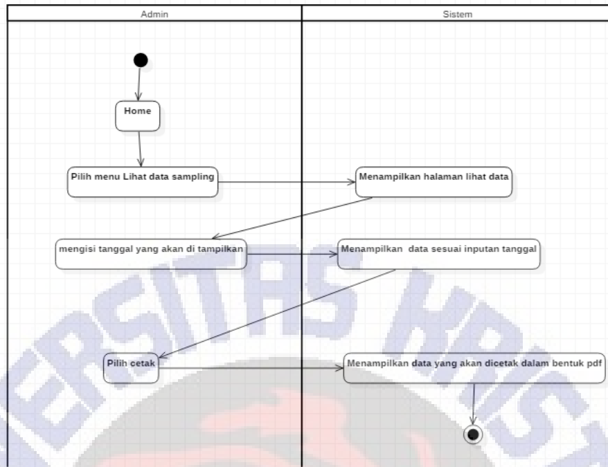
Activity diagram proses lihat data dan cetak bukti sampling
