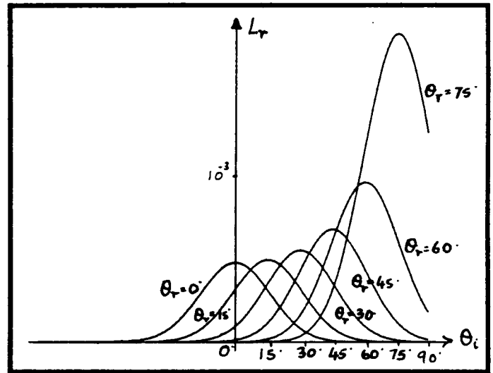
(d) \sigma_\alpha = 7.99
