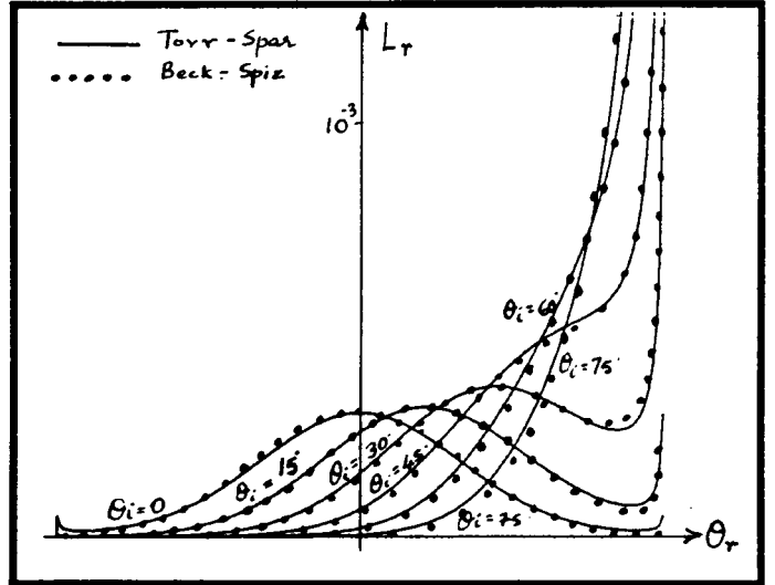
(d) \sigma_\alpha = 13.0
