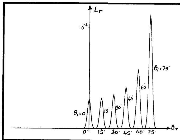
(d) \sigma_\alpha = 1.0
