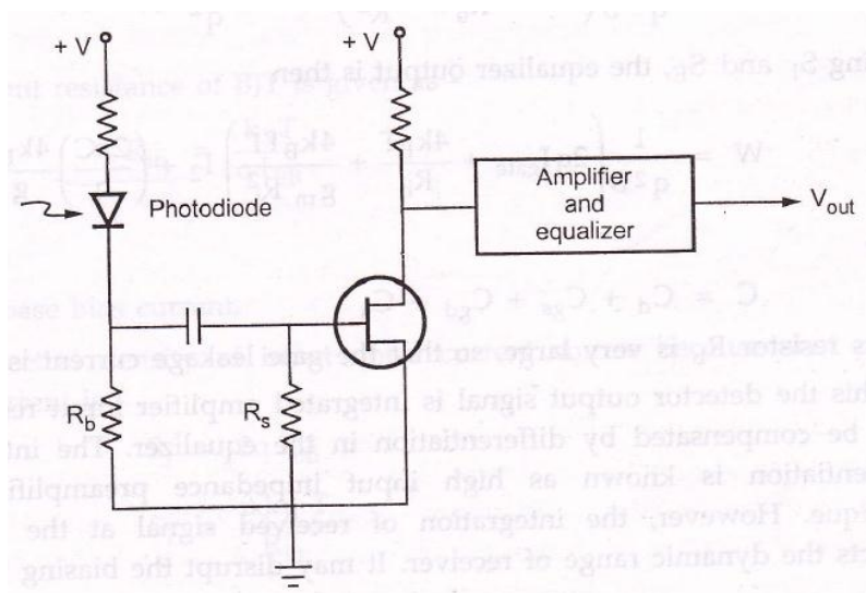
Fig. 5.1.5 High input impedance preamplifier using FET
