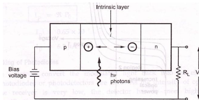
Fig. 3.2.2 PIN photodiode
