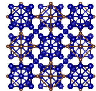
Cr 23 C 6
