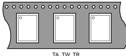
Figure 43. WLCSP 3-, 4-, 6-, 8-, 10-, & 12-Bump
