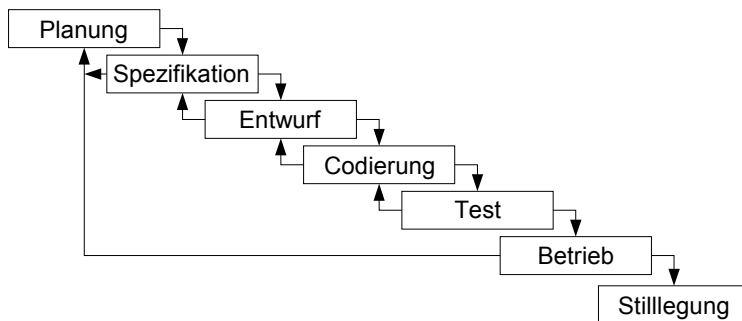
Abbildung 1.1 Software-Lebenszyklus
