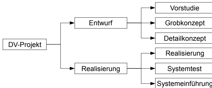
Abbildung 1.2 Das 6-Phasenmodell
