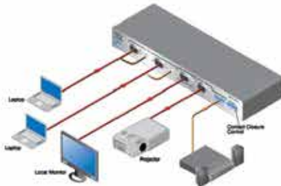
AV Switches
