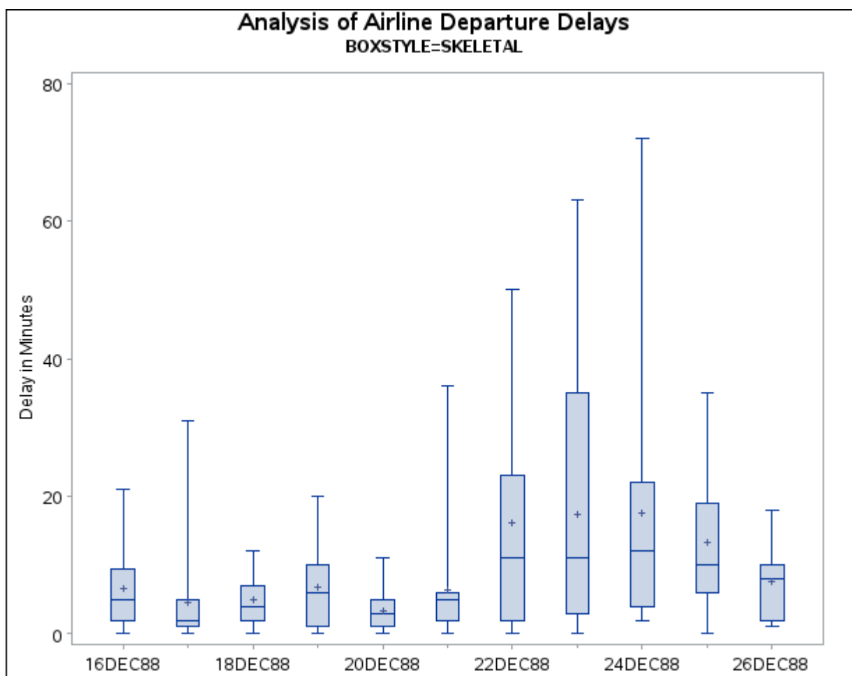
Output 28.3.1 BOXSTYLE=SKELETAL
