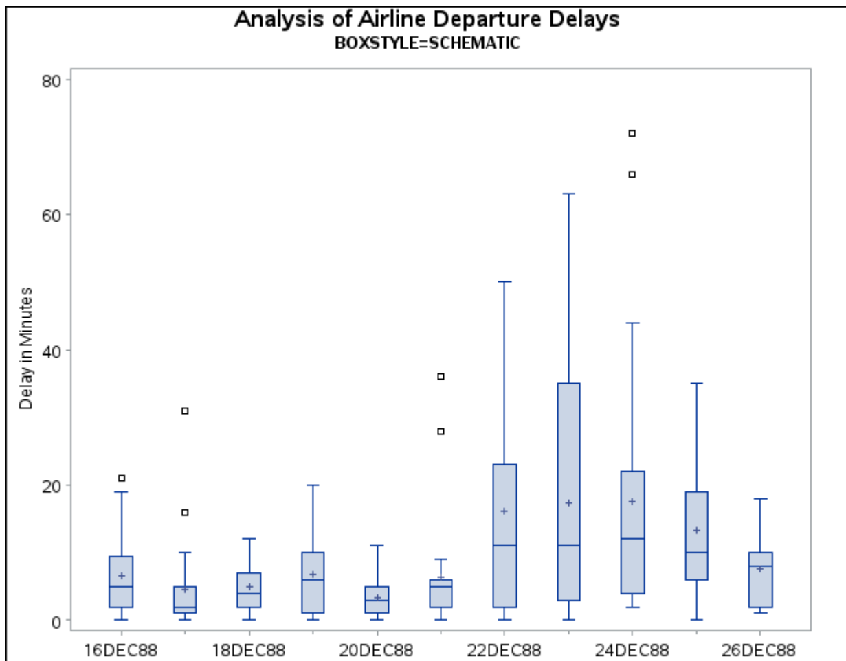
Output 28.3.2 BOXSTYLE=SCHEMATIC
