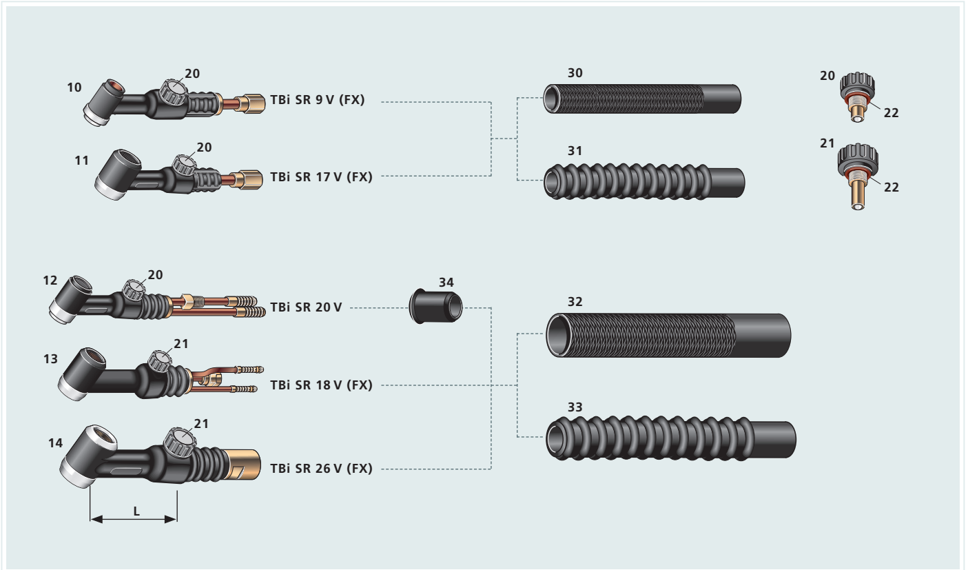
Empuñaduras en tubo para antorchas con válvula / Handle tubes for torch bodies with valve
